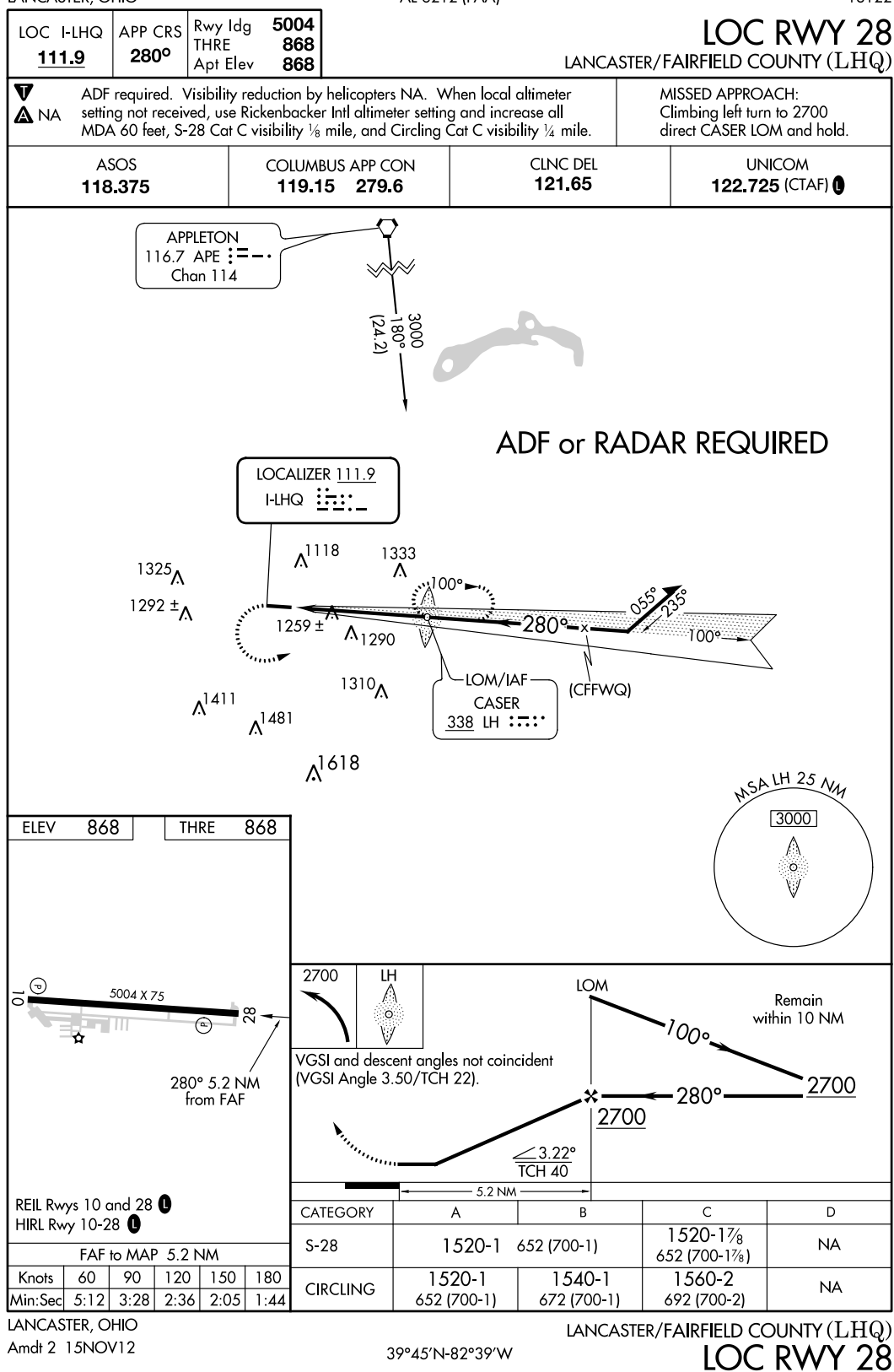
FIGURE 239.—LOC RWY 28 (LHQ).
