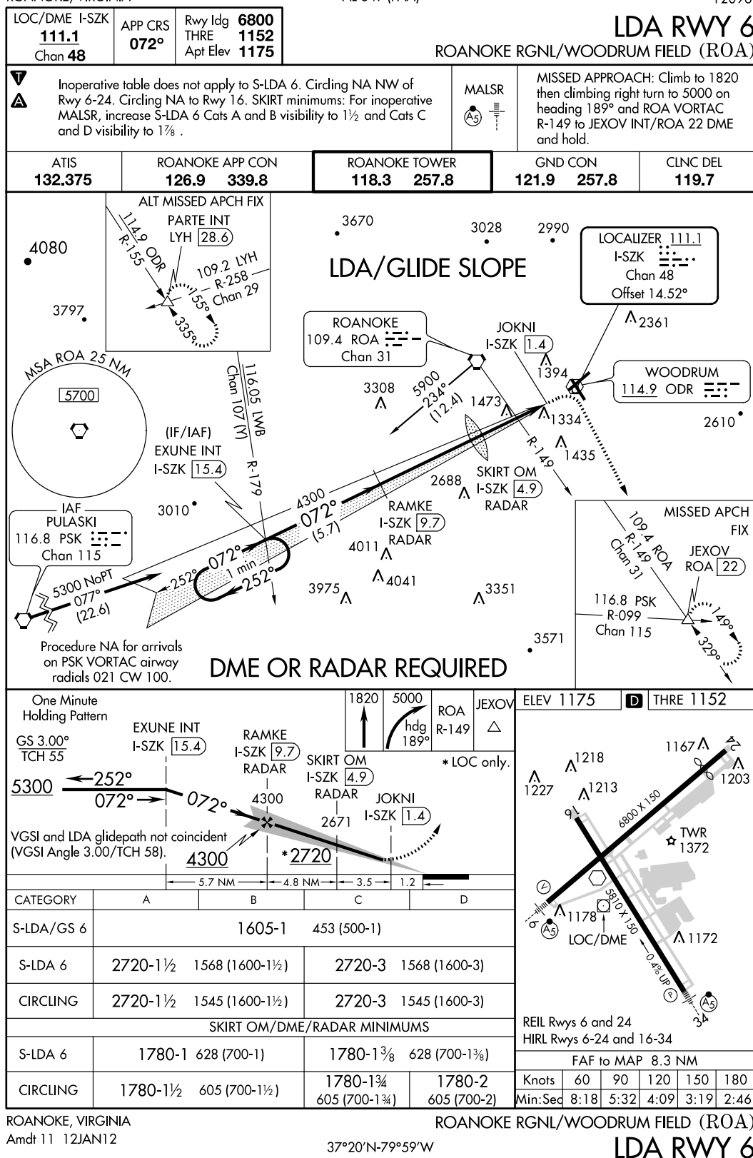
FIGURE 244.—LDA RWY 6 (ROA).
