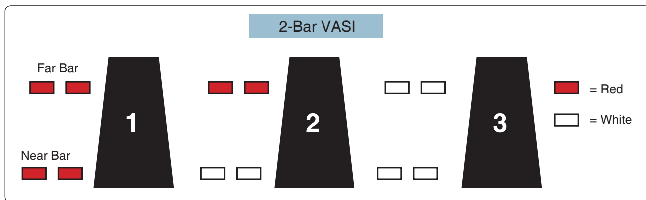
FIGURE 134.—2-BAR VASI.
