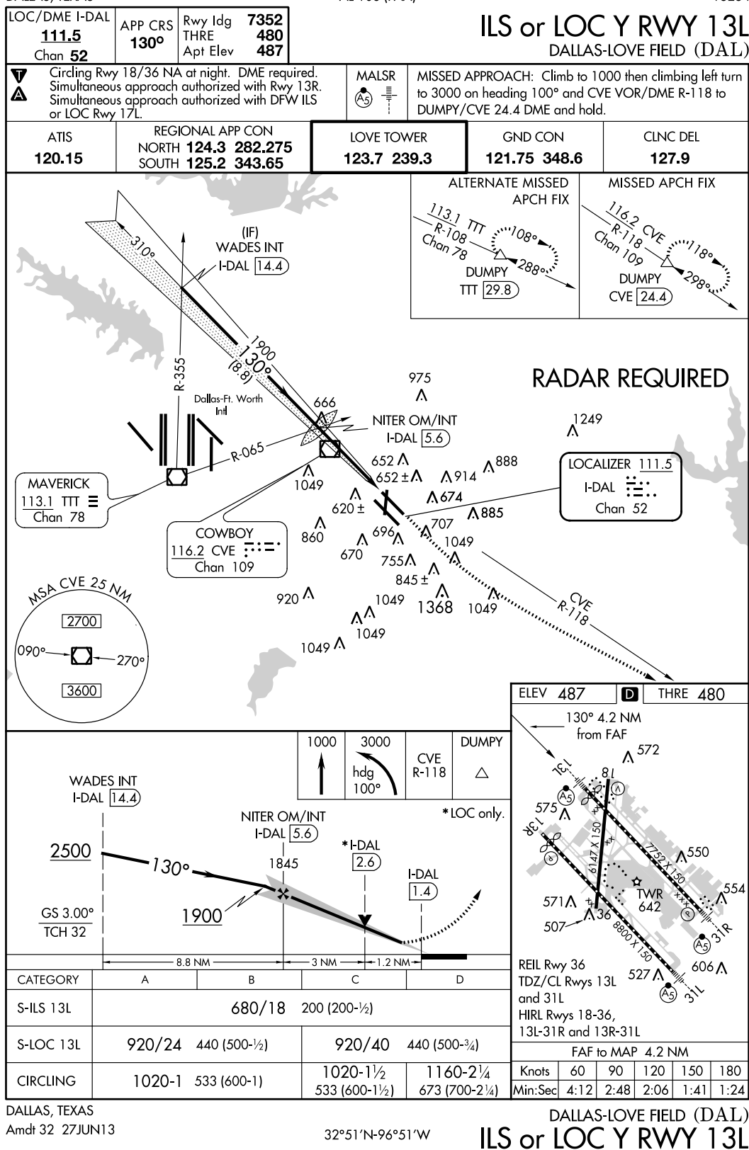
FIGURE 178.—ILS or LOC Y RWY 13L (DAL).
